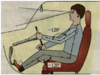
Рис. 1. Регулировка сиденья водителя
