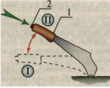
Рис. 30. Рычаг стояночного тормоза: 1 - рычаг стояночного тормоза; 2 - кнопка фиксатора рычага
