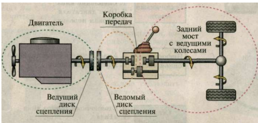
Рис. 25. Схема силовой установки автомобиля на примере заднеприводного автомобиля
