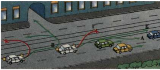
Рис. 114. Маневрирование на дороге с трамвайными путями
