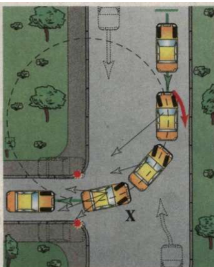
Рис. 151. Въезд в «боксы» задним ходом налево
