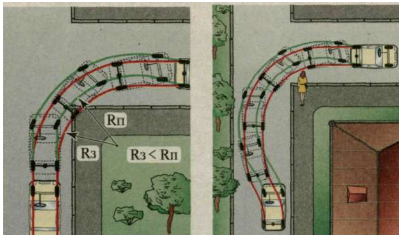
Рис. 54. Наезд на угол тротуара
