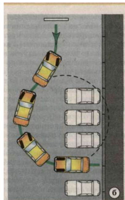
Рис. 148. Въезд в «боксы» задним ходом направо: а) с «кругом», значительно смещенным влево; б) с «петлей» во время движения задним ходом; в) совмещенный с разворотом в три приема
