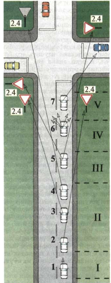
Рис. 101. Определение главенства дорог
