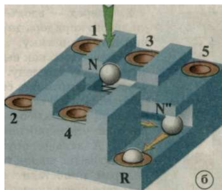
Рис. 22. Передача заднего хода: а) слева; б) справа
