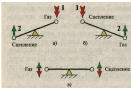
Рис. 34. «Качели»
