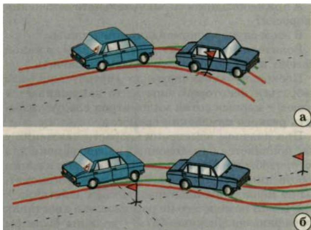
Рис. 42. Траектории движения передних и задних колес
