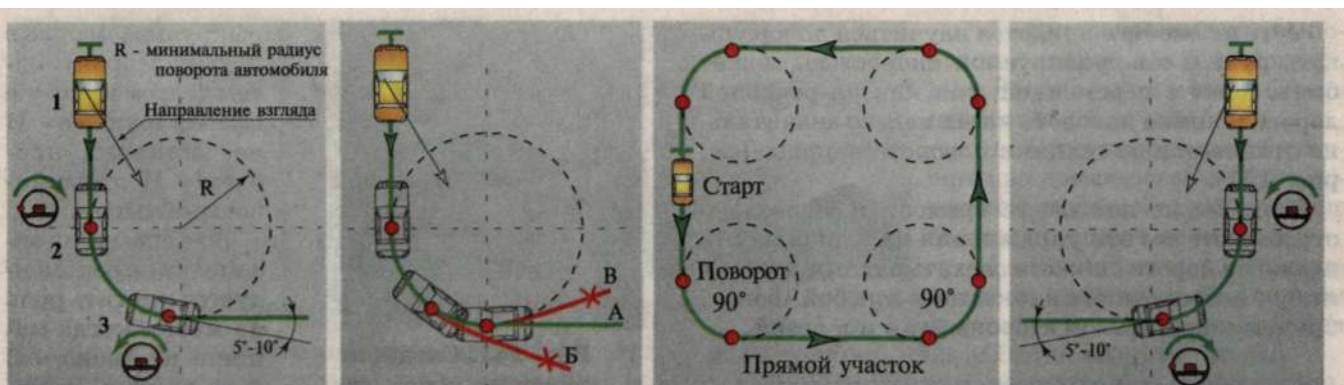
Рис. 136. Поворот назад под углом 90^\circ направо
