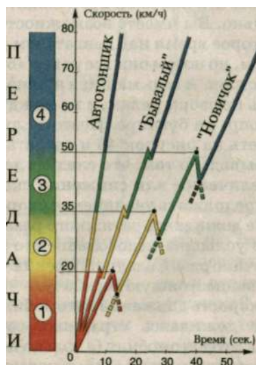
Рис. 43. Соответствие скорости и передачи
