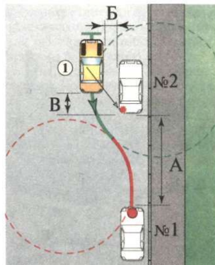
Рис. 152. Планирование места остановки и последующей траектории движения
