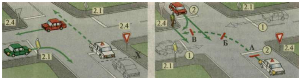
Рис. 100. Поворот налево со второстепенной дороги на главную
