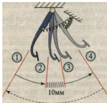
Рис. 32. Положения педали сцепления
