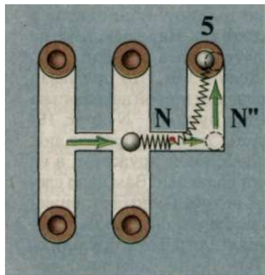
Рис. 21. Пятая передача
