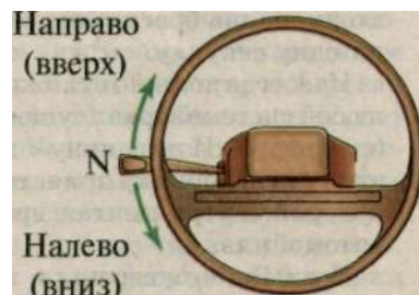
Рис. 29. Рычаг переключения указателей поворота
