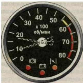
Рис. 31. Тахометр
