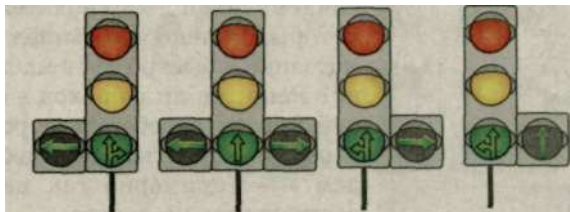
Рис. 98. Варианты дополнительных секций светофора
