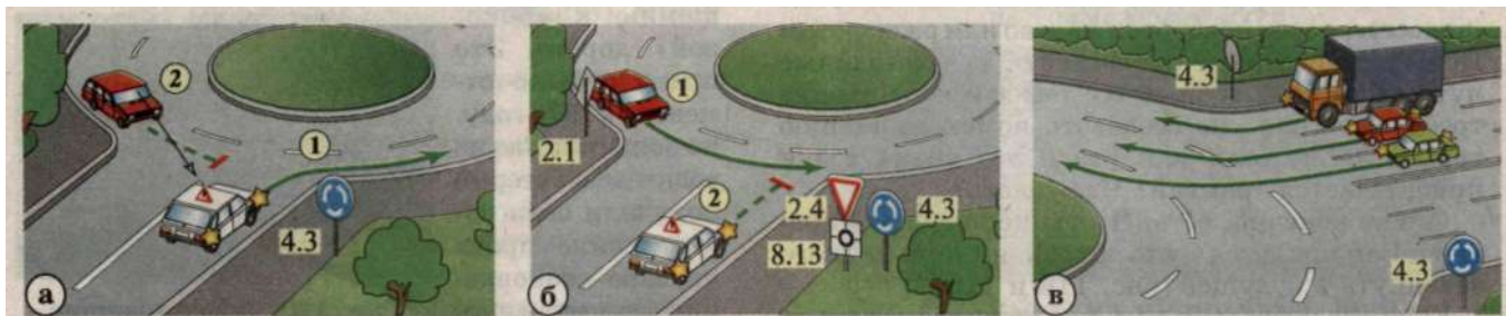
Рис. 121. Въезд на «круг»
