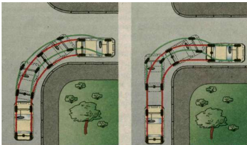
Рис. 52. Плавная траектория Рис. 53. «Ломаная» траектория
