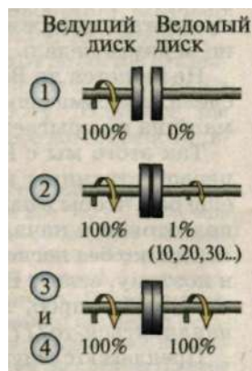
Рис. 33. Положения дисков сцепления
